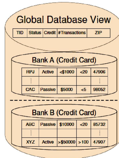
Fig.1. Database partitioning
